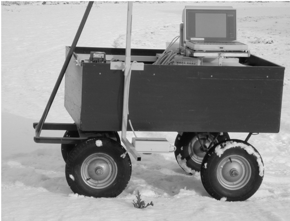
Bild 5: Messwagen für die Erfassung der Reflexion verschiedener Pflanzen auf dem Feld
