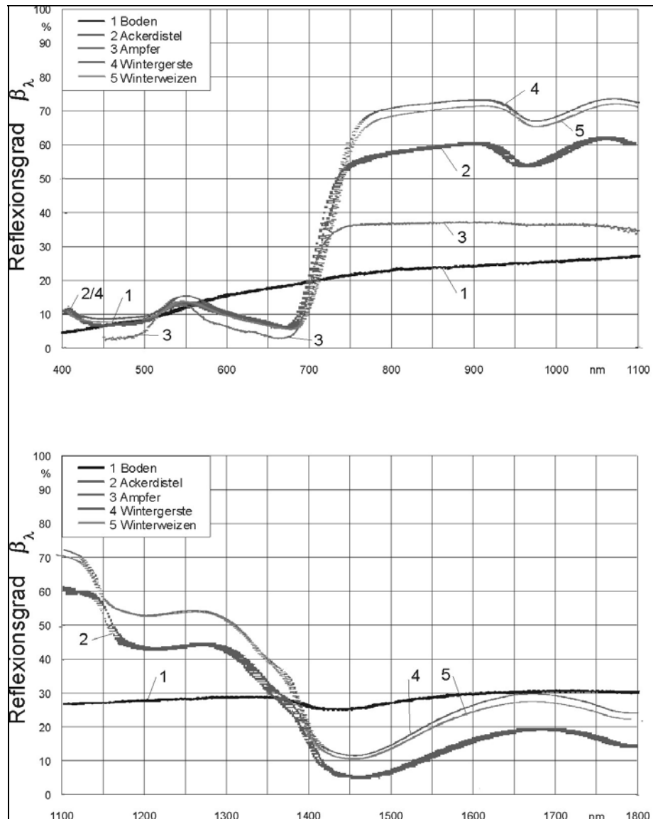
Bild 6: Reflexion von Boden, Wintergetreide, Ampfer und Ackerdistel im Wellenlängenbereich des Umgebungslichtes zwischen 400 nm und 1800 nm
