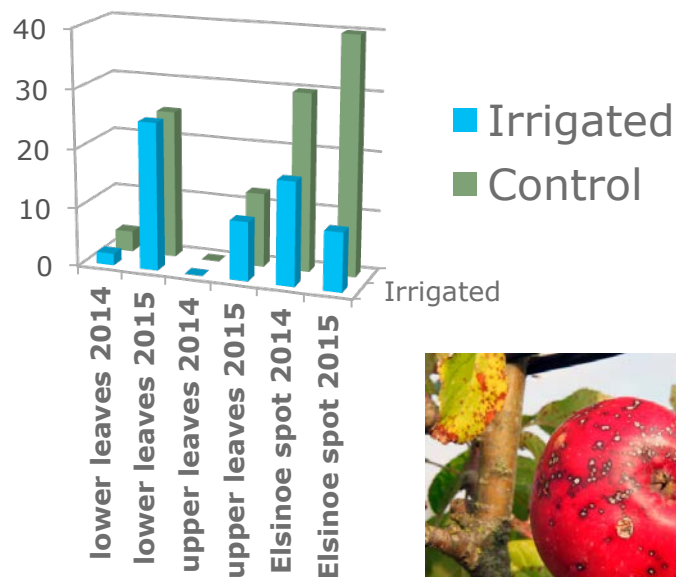
Median % blade med skurv og æbleøjeplet i 'Collina'
