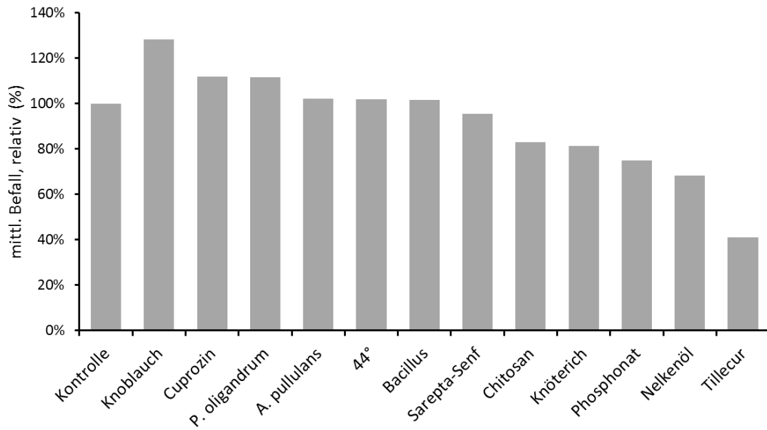
Abb. 2. Beizung - Lagerversuch: Mittlerer Knollenbefall (in %, relativ zur unbehandelten Kontrolle) nach künstlicher Inokulation, Beizung und 6-wöchiger Inkubation bei 15°C. Mittelwerte aus 6 Einzelversuchen mit je n = 10 oder 30 Knollen.
