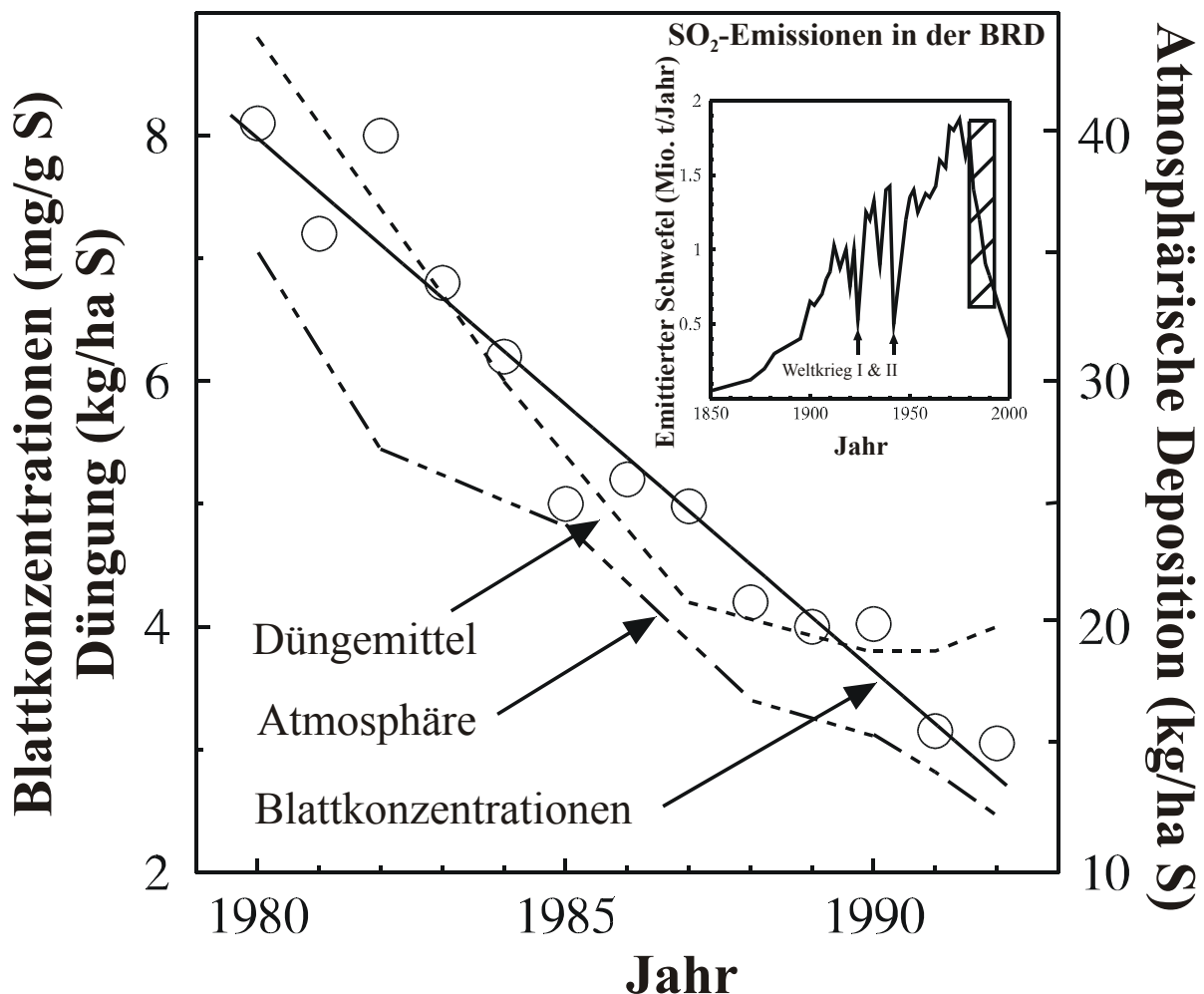
Abb. 2: Entwicklung der Einträge an atmosphärischem SO 2 -S, Anwendung S-enhaltender Dünger und S-Gehalten in Blättern von Raps ( Brassica napus ) in Norddeutschland (SCHNUG und HANEKLAUS 1994)
