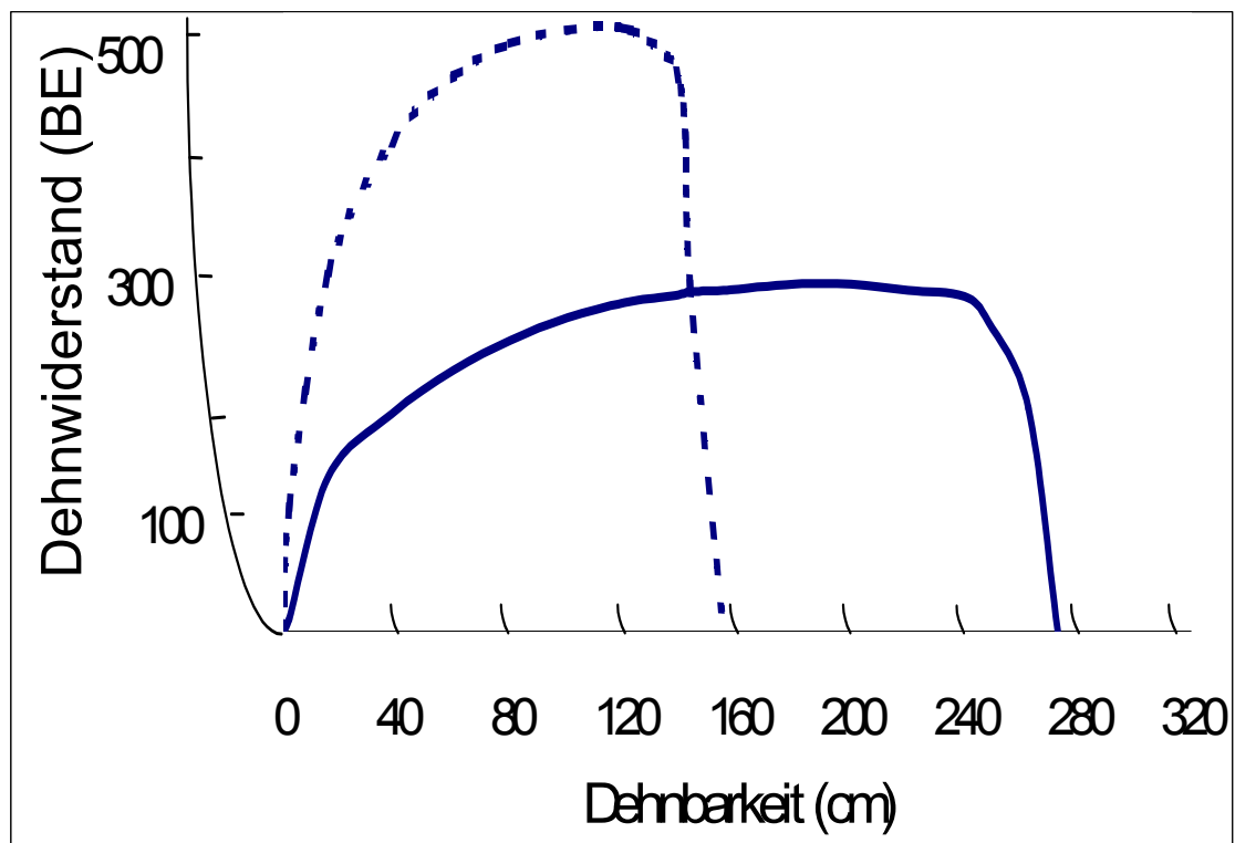
Abb. 1: Extensogrammkurven für Mehle (Sorte OLYMPIC) mit unterschiedlichen Schwefelgehalten. Kontrolle (—): 0,146 % S, 1,82 % N, N:S-Verhältnis: 12,5. Mehl mit niedrigem S-Gehalt (- - - -): 0,089 % S, 1,72 % N, N:S-Verhältnis: 19,3 (WRIGLEY et al. 1984)
