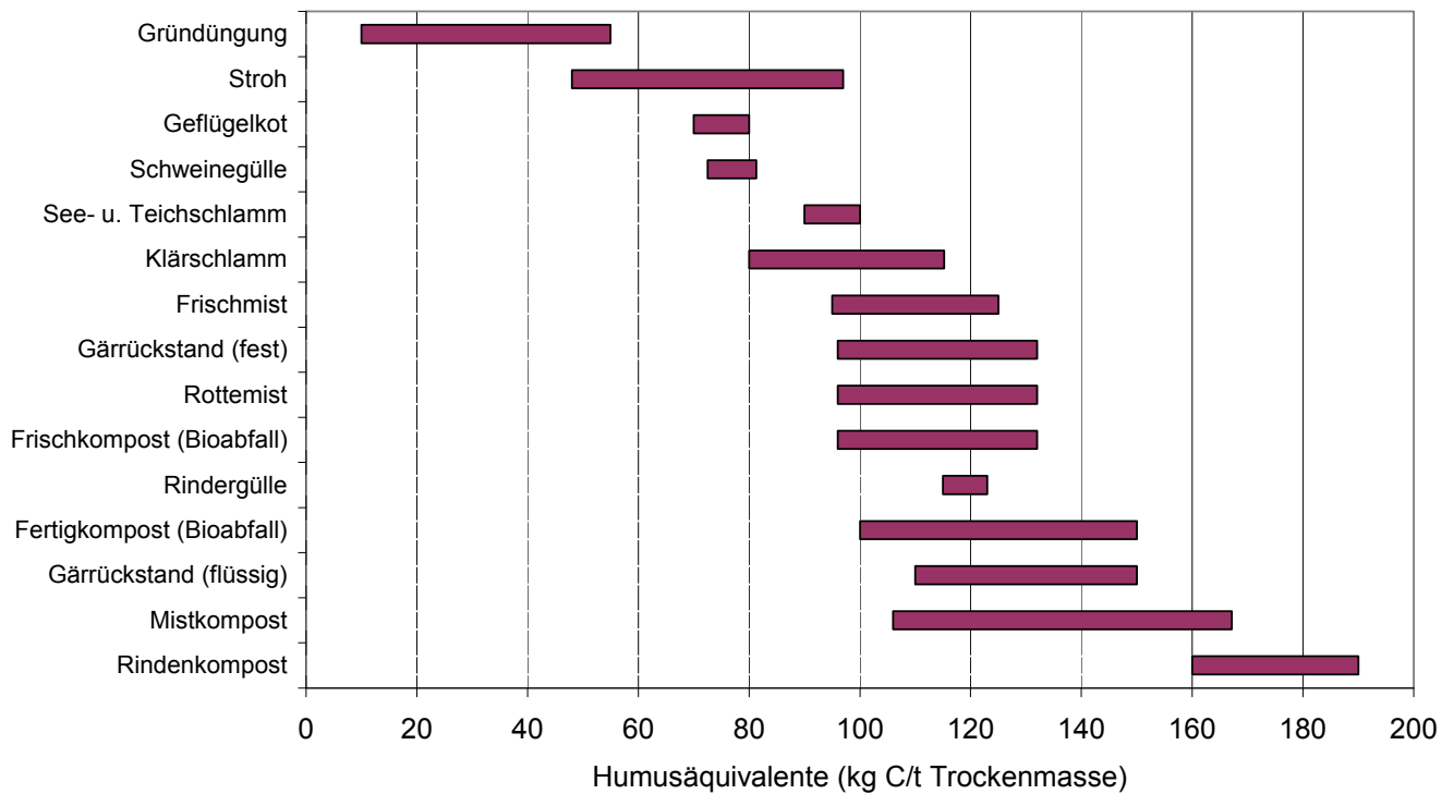
Abbildung 6: Humifizierungskoeffizienten der organischen Materialien in der STAND-Methode, berechnet nach Frischmasse (oben) und Trockenmasse (unten)
