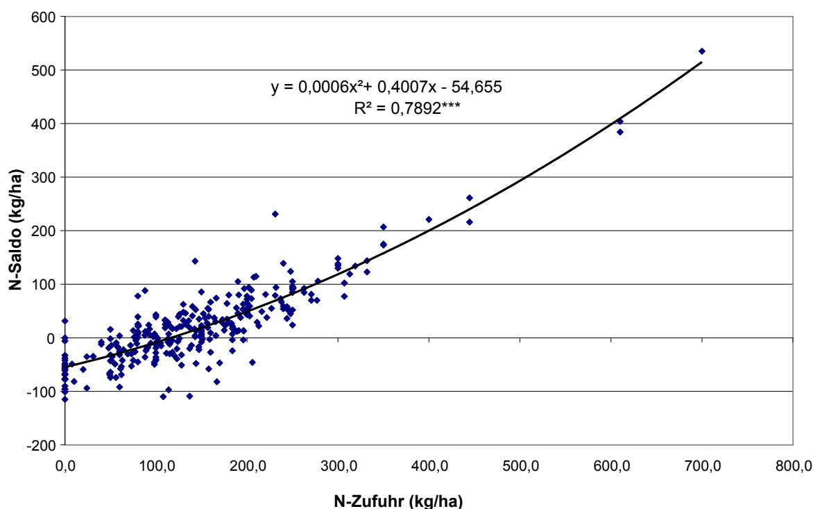
Abbildung 29: Beziehung zwischen Gesamt-N-Zufuhr und N-Saldo aus 39 Dauerversuchen (ohne Berücksichtigung der N-Herkünfte aus Deposition, N_T -Saldo Boden und N-Zufuhr aus dem Untergrund)
