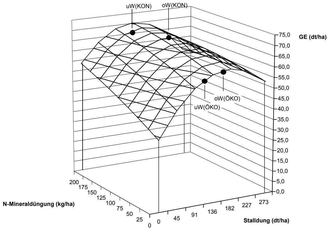
Abbildung 16: Zusammenhang zwischen steigender Zufuhr an N-Mineraldüngung und Stallung auf die Getreideeinheiten (GE) in einem Dauerdüngungsversuch aus Groß Kreutz (siehe KOLBE & PRUTZER 2004) sowie Einordnung von Optimalvarianten (100 % Bedarfsdeckung an organischer Substanz), ermittelt mit den unteren (uW) und oberen Werten (oW) der LUFA-Methode im konventionellen (KON) und ökologischen (ÖKO) Bewirtschaftungssystem
