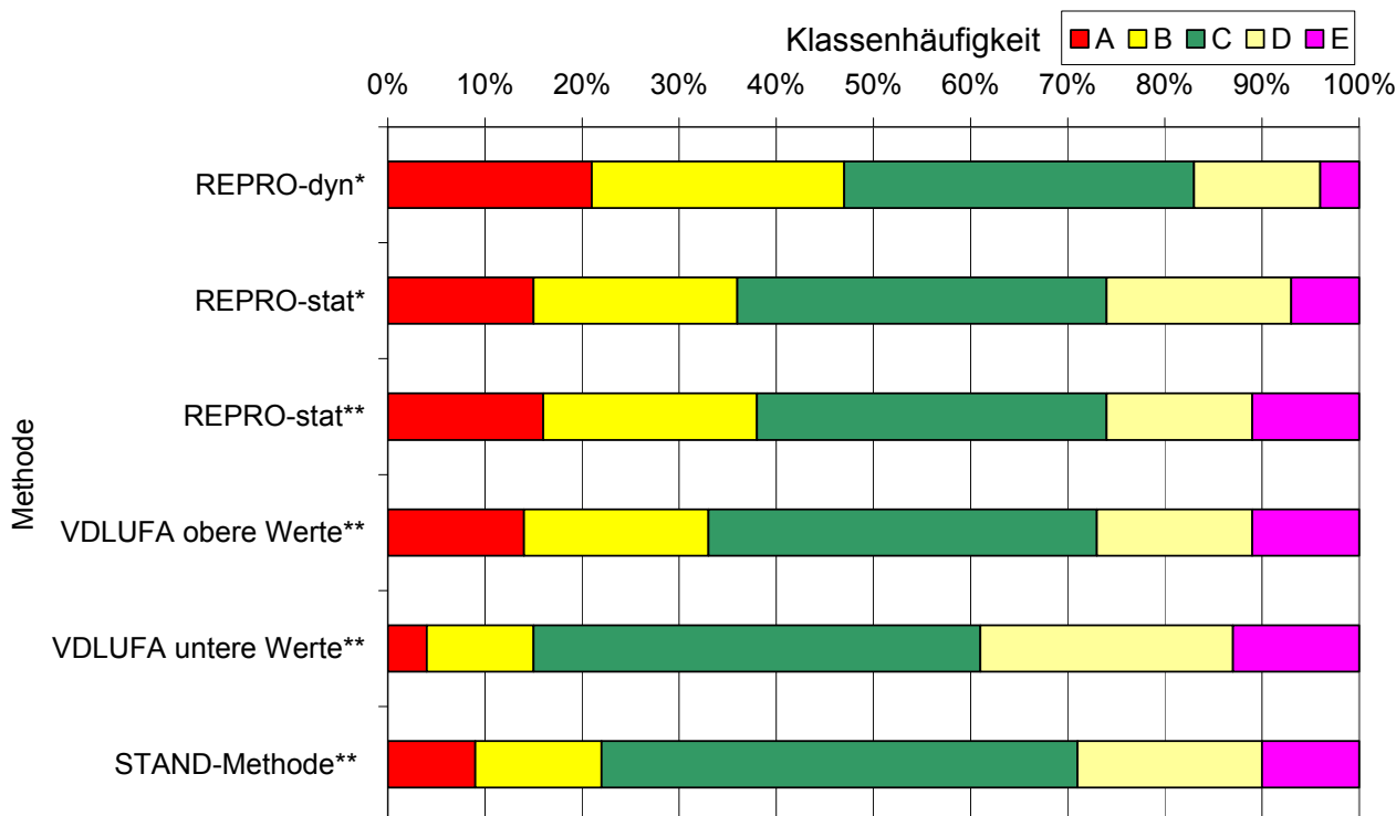
Abbildung 2: Klassenhäufigkeiten (in %) der Humusversorgung der Dauertestflächen in Sachsen nach verschiedenen Bilanzierungsmethoden (* 1.058 Flächen nach MÖNISCHE et al. 2005; ** 760 Flächen nach SEIBT 2007)
