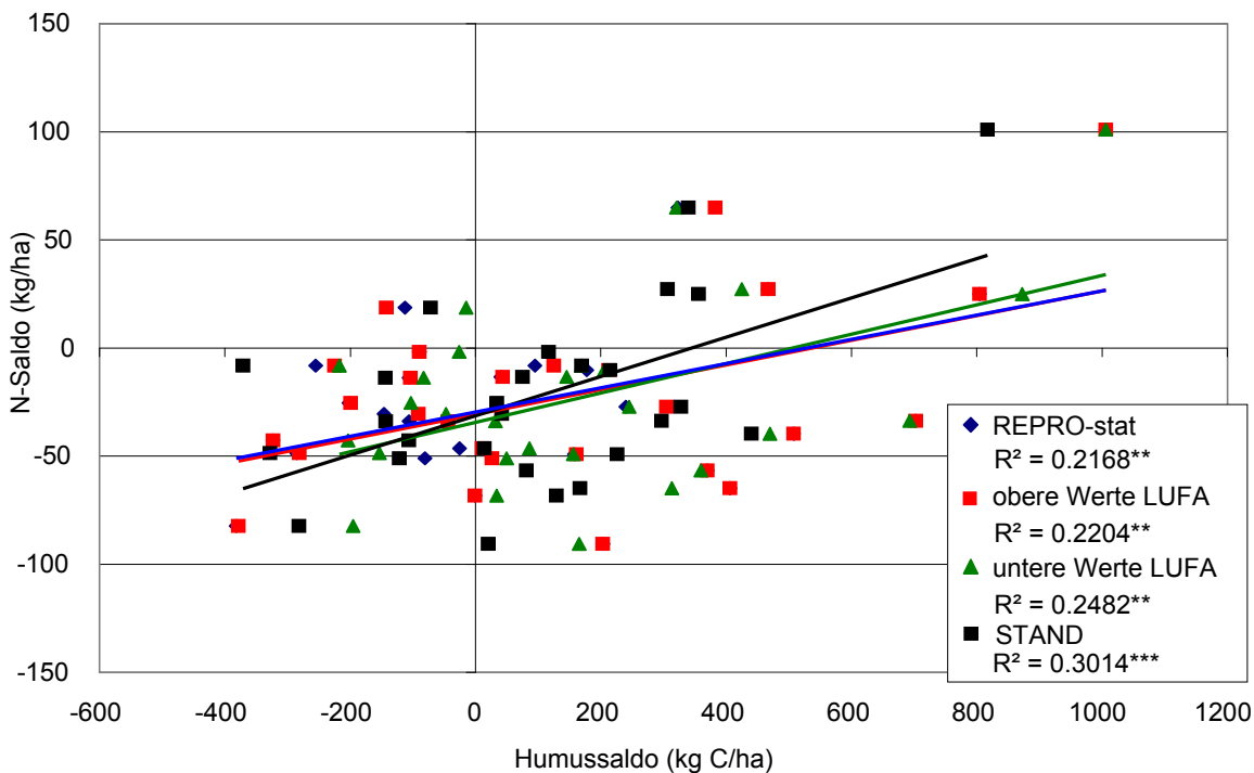
Abbildung 24: Zusammenhang zwischen den mit verschiedenen Methoden ermittelten Humussalden und den N-Salden, ermittelt in den Studien von BROCK et al. (2008) (oben) sowie den DTF in Sachsen (SEIBT 2007) (unten)
