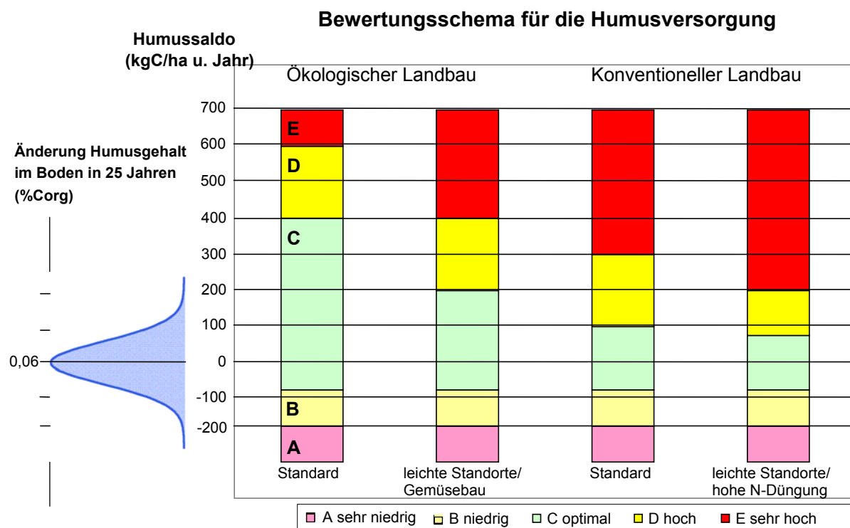
Abbildung 3: Versorgungsgruppen für Humus für den konventionellen und ökologischen Landbau (KOLBE 2007b)
