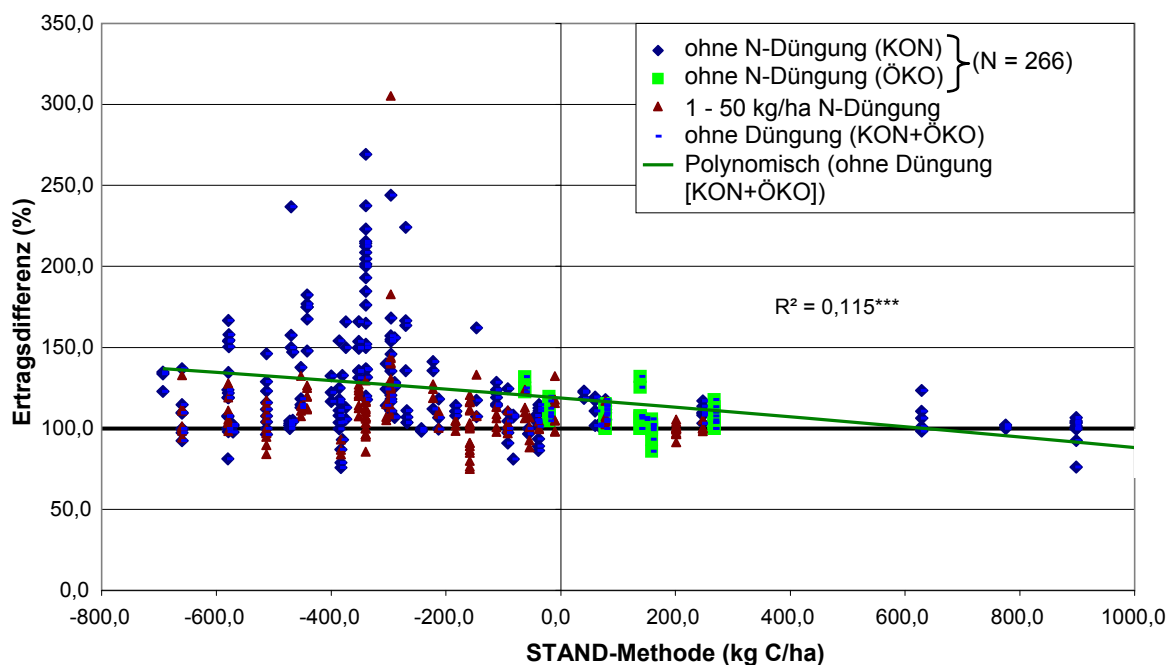
Abbildung 14: Einfluss unterschiedlicher Versorgungs-niveaus (Standard) mit organischer Substanz entsprechend den unteren Werten (oben) der LUFA-Methode sowie der standortangepassten Methode (unten) auf die mittlere Ertragsdifferenz der Fruchtarten jeweils ermittelt nach einer zusätzlichen Zufuhr an organischer Substanz in Abhängigkeit von den extensiven konventionellen (KON) und den ökologischen Varianten (ÖKO) aus 39 Dauerversuchen (A- E-Grenzen der Versorgungsgruppen siehe Abb. 3)
