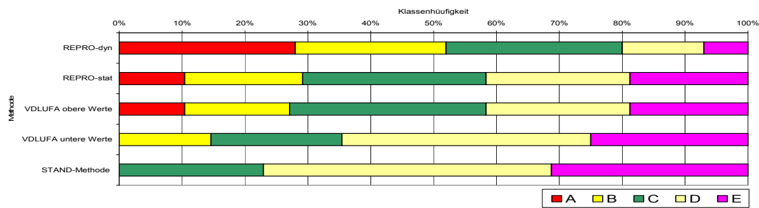
Abbildung 4: Klassenhäufigkeiten (in %) der Humusversorgung der einzelnen Agrarstrukturgebiete in Sachsen, ermittelt mit verschiedenen Humusbilanzmethoden
