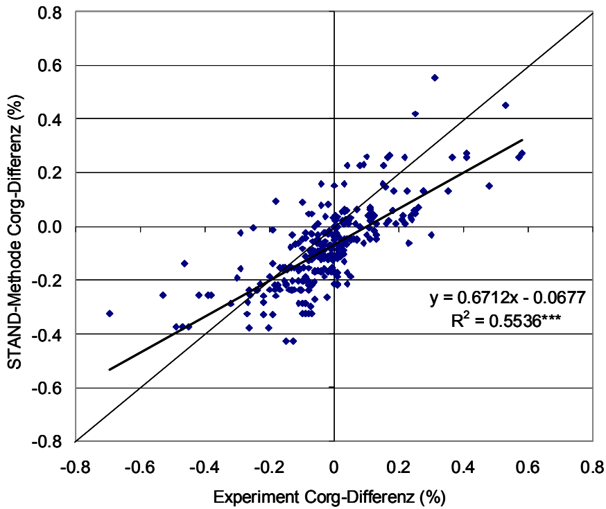
Abbildung 8: Beziehung zwischen den experimentell ermittelten C_{org} -Differenzen der Dauerversuche und den mit der STAND-Methode berechneten Werten, ermittelt anhand von Ergebnissen aus 39 Dauerversuchen
